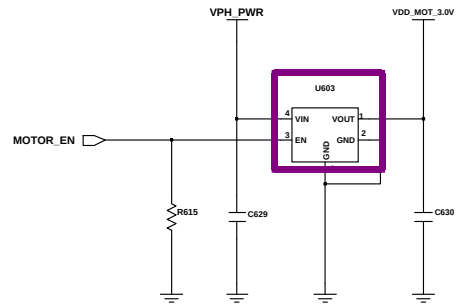
MOTOR LDO(150mA)
